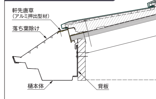
横葺き屋根
